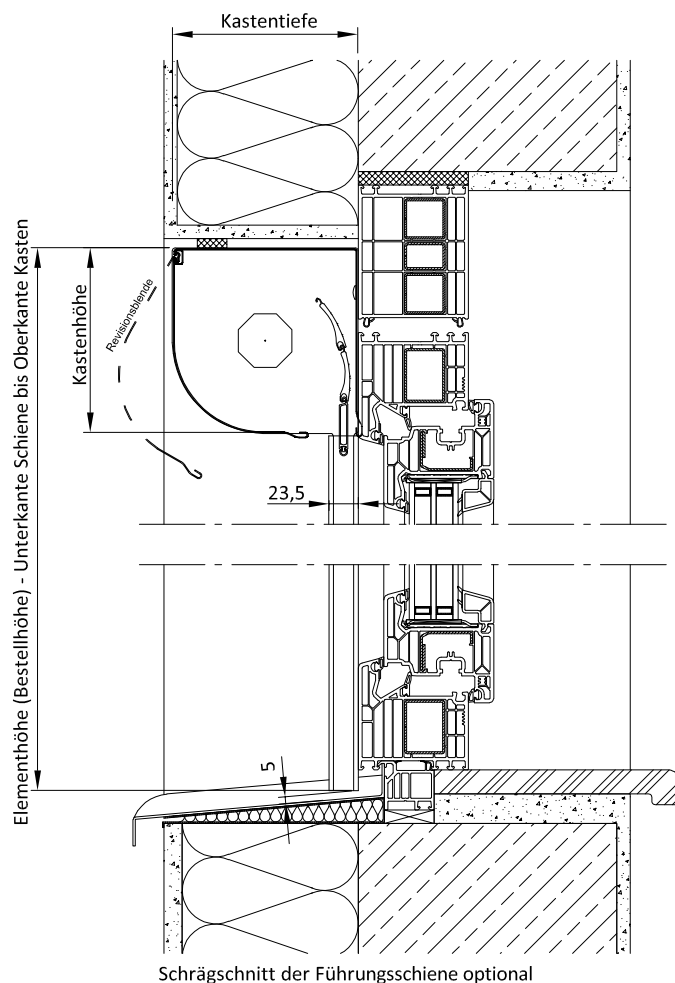
Schrägschnitt der Führungsschiene optional
