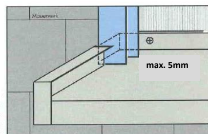
Bild 2 Auslenkung des Bordprofils für den Einbau der Rollladenführungsschiene (in unverputztem/ungedämmtem Zustand, Isometrie)
